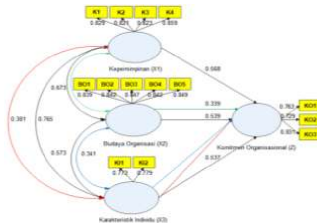
Gambar 4. Analisis Jalur Model Penelitian Keseluruhan
